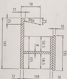
SEC-B-B SCALE-1:2
